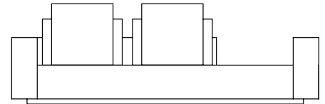
SOFA 300 x 110 x 65cm (LxPxA) Almofadas: 02 unidades decorativa 60x60cm 02 unidades de encosto (L=78cm)
