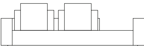
SOFA 320 x 110 x 65cm (LxPxA) Almofadas: 02 unidades decorativa 60x60cm 02 unidades de encosto (L=88cm)
