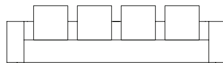
SOFA 320 x 080 x 65cm (LxPxA) Almofadas: 04 unidades pastel 50x50cm
