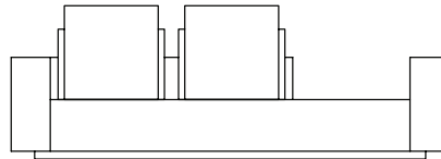
SOFA 280 x 110 x 65cm (LxPxA) Almofadas: 02 unidades decorativa 60x60cm 02 unidades de encosto (L=70cm)
