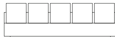
SOFA 280 x 080 x 65cm (LxPxA) Almofadas: 05 unidades pastel 50x50cm
