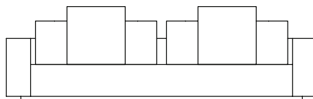
SOFA 320 x 110 x 65cm (LxPxA) Almofadas: 02 unidades decorativa 60x60cm 02 unidades de encosto (L=125cm)
