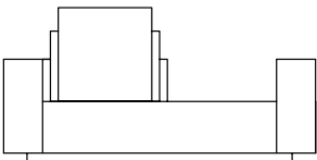
SOFA 200 x 110 x 65cm (LxPxA) Almofadas: 01 unidade decorativa 60x60cm 01 unidade de encosto (L=70cm)
