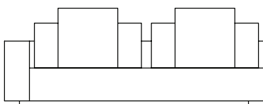
SOFA 260 x 110 x 65cm (LxPxA) Almofadas: 02 unidades decorativa 60x60cm 02 unidades de encosto (L=108cm)
