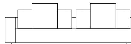
SOFA 300 x 110 x 65cm (LxPxA) Almofadas: 02 unidades decorativa 60x60cm 02 unidades de encosto (L=127cm)
