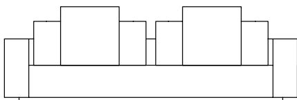
SOFA 300 x 110 x 65cm (LxPxA) Almofadas: 02 unidades decorativa 60x60cm 02 unidades de encosto (L=115cm)
