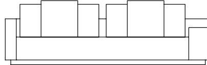
SOFÁ 280 X 100 X 63cm (LxPxA) Almofadas: 02 unidade decorativa 60x60 com faixa 02 unidades de encosto 02 unidades rolinho de encosto (L=120cm)
