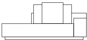
SOFÁ 200 X 100 X 63cm (LxPxA) Almofadas: 01 unidade decorativa 60x60cm com faixa 01 unidade de encosto (L=90cm) 01 unidade rolinho de encosto
