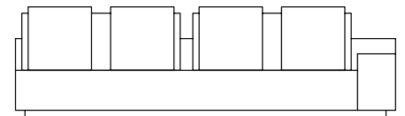
SOFÁ 300 X 100 X 63cm (LxPxA) Almofadas: 04 unidades decorativa 60x60cm com faixa 02 unidades de encosto (L=125cm) 02 unidades rolinho de encosto
