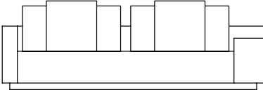
SOFÁ 260 X 100 X 63cm (LxPxA) Almofadas: 02 unidade decorativa 60x60 com faixa 02 unidades de encosto 02 unidades rolinho de encosto (L=110cm)
