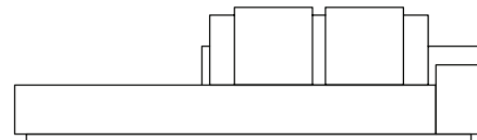
SOFÁ 300 X 100 X 63cm (LxPxA) Almofadas: 04 unidades decorativa 60x60cm com faixa 01 unidade de encosto (L=140cm) 01 unidade rolinho de encosto
