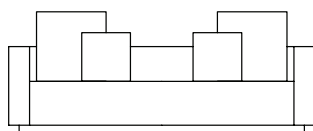
SOFÁ 220 X 160 X 63cm (LxPxA) Almofadas: 02 unidades decorativa 60x60cm com faixa 02 unidades decorativa 100x100cm
