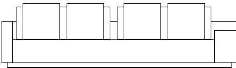
SOFÁ 320 X 100 X 63cm (LxPxA) Almofadas: 03 unidade decorativa 60x60 com faixa 03 unidades de encosto 03 unidades rolinho de encosto (L=90cm)
