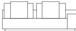
SOFÁ 220 X 100 X 63cm (LxPxA) Almofadas: 02 unidades decorativa 60x60cm com faixa 02 unidades de encosto (L=85cm) 02 unidades rolinho de encosto
