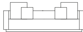
SOFÁ 240 X 130 X 63cm (LxPxA) Almofadas: 02 unidades decorativa 60x60cm com faixa 02 unidades decorativa 100x100cm
