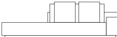
SOFÁ 280 X 100 X 63cm (LxPxA) Almofadas: 02 unidades decorativa 60x60cm com faixa 01 unidade de encosto (L=130cm) 01 unidade rolinho de encosto
