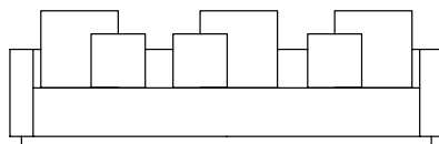
SOFÁ 280 X 130 X 63cm (LxPxA) Almofadas: 03 unidades decorativa 60x60cm com faixa 03 unidades decorativa 100x100cm
