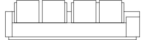
SOFÁ 300 X 100 X 63cm (LxPxA) Almofadas: 03 unidade decorativa 60x60 com faixa 03 unidades de encosto 03 unidades rolinho de encosto (L=83cm)
